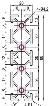
NFS5-2080 HFS5-2080
