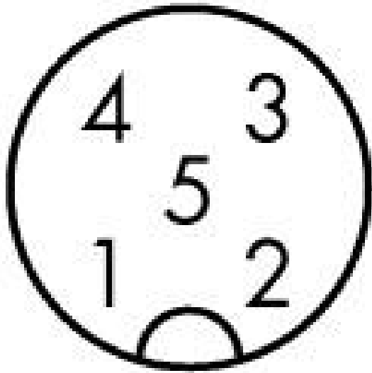
M12-Stecker
